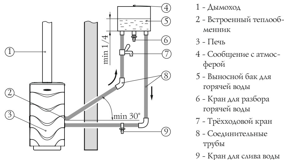
Рисунок 14. Схема монтажа системы водонагрева с использованием встроенного теплообменника
