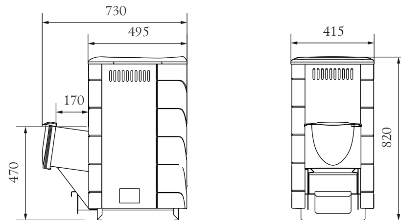
Рисунок 5. Габаритно-монтажные размеры печи «Тунгуска 2017 Carbon»
