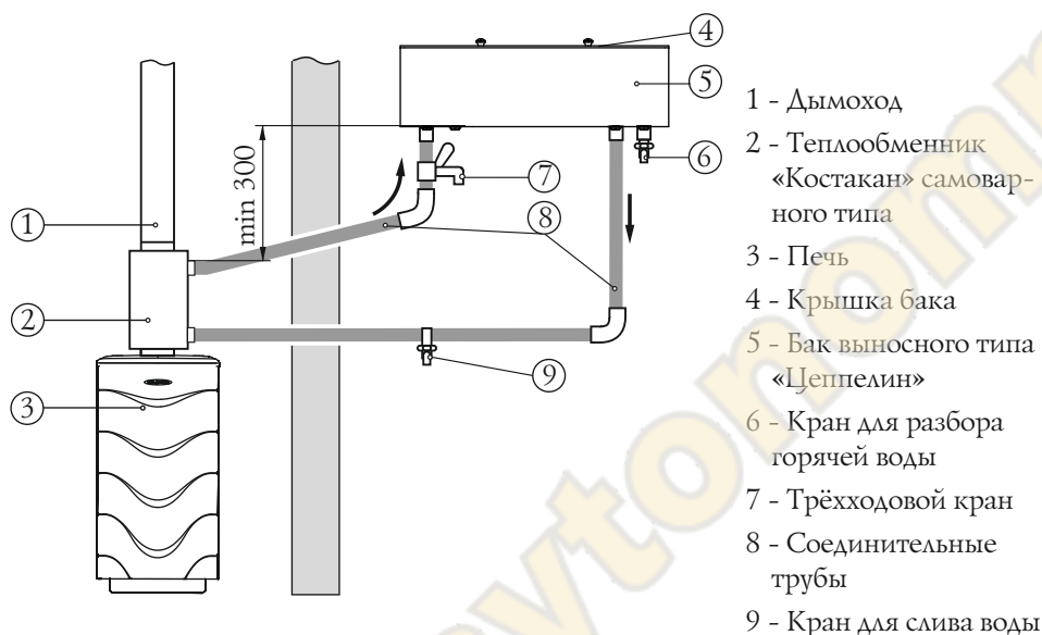
Рисунок 15. Схема монтажа системы водонагрева с использованием теплообменника «самоварного» типа
