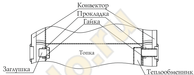
Рисунок 13. Демонтаж теплообменника.
