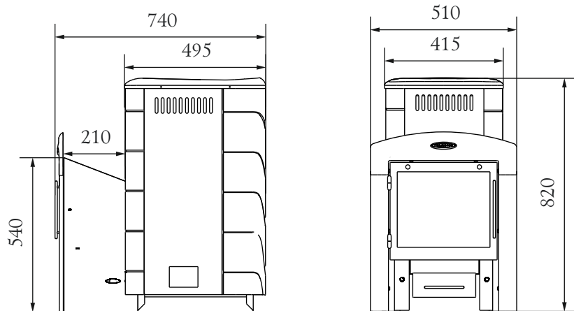
Рисунок 6. Габаритно-монтажные размеры печи «Тунгуска 2017 Carbon Витра»
