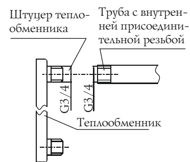
Рисунок 16. Присоединение трубопровода напрямую.
