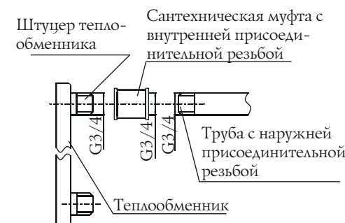
Рисунок 17. Присоединение трубопровода через муфту.
