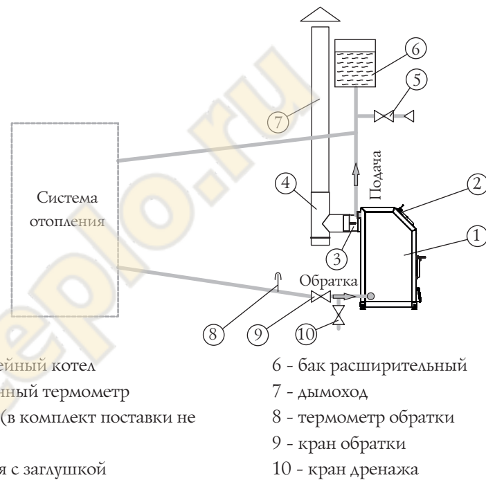
Рисунок 10. Подключение открытой системы отопления с естественной циркуляцией.
