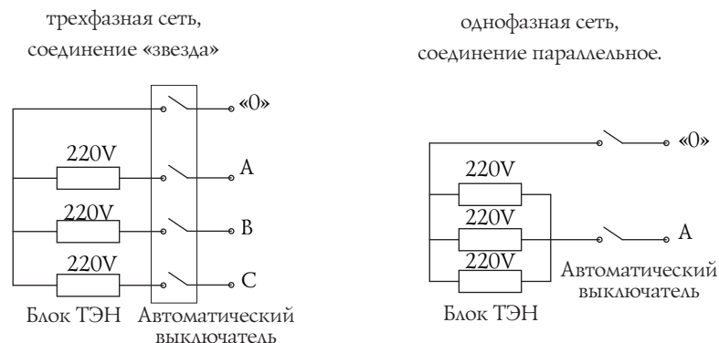
Рисунок 13. Схемы соединения блока ТЭН.
