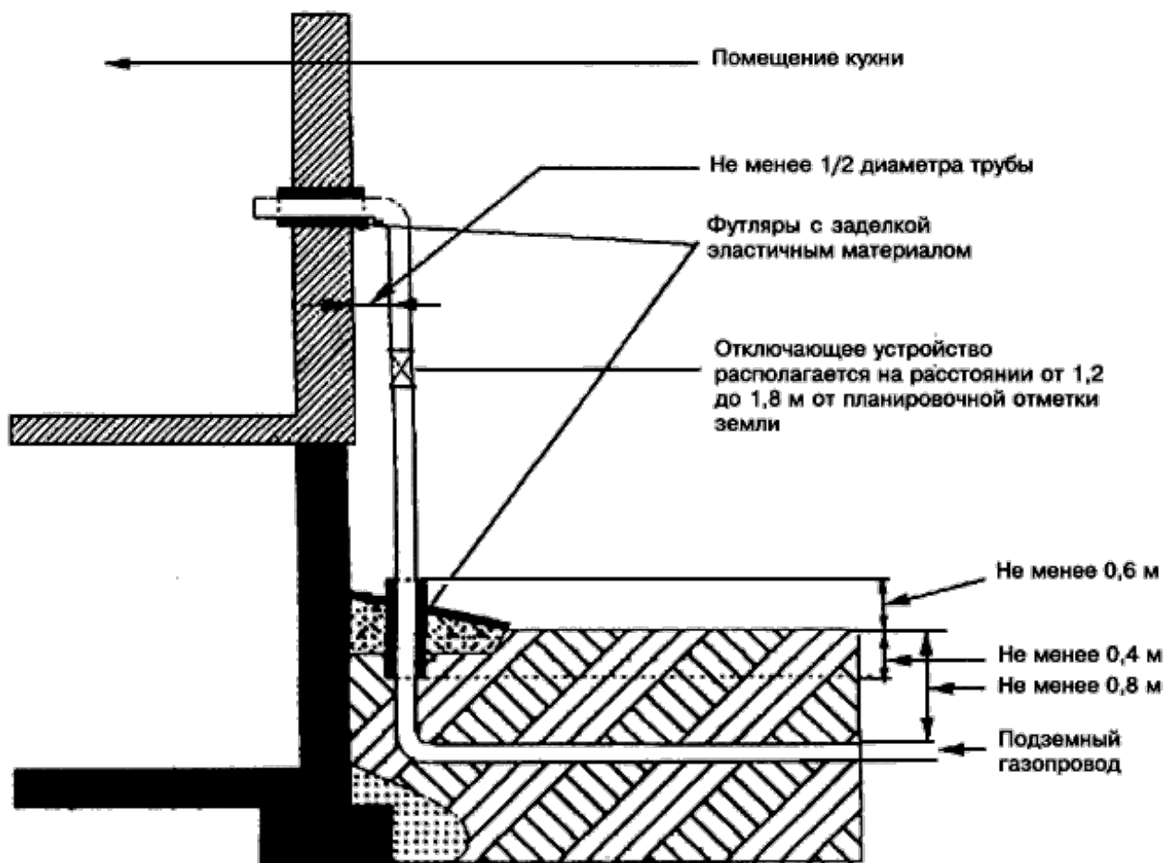
Рисунок 9.1 - Газовый ввод
