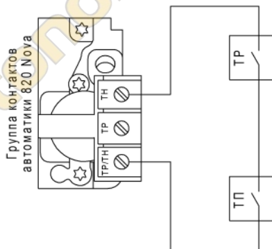
Схема энергозависимого котла с автоматикой SIT820 NOVA
