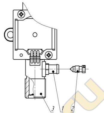
1 – патрубок замера давления газа; 2 – винт с уплотнением; 3 – входной патрубок газового узла.
