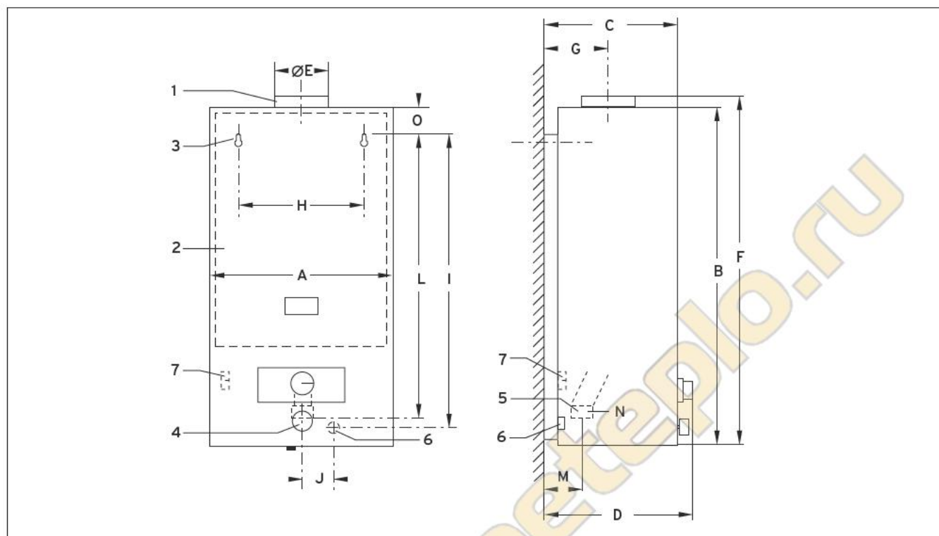
Рис. 4.1 Размеры
