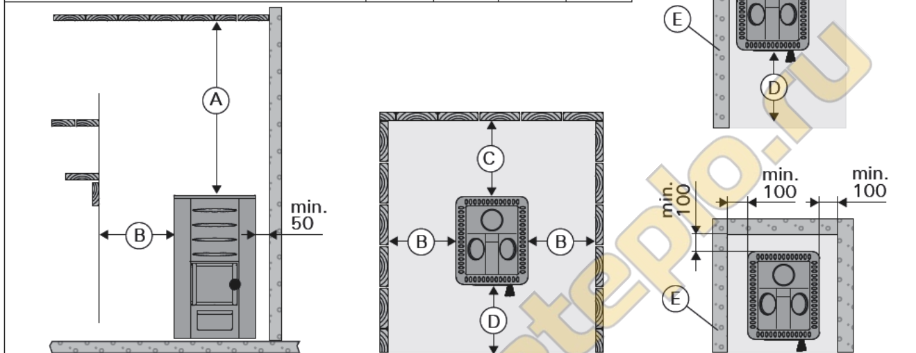
Рисунок 7. Безопасные расстояния (все размеры приведены в миллиметрах)
