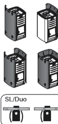
Рисунок 8. Безопасные расстояния с защитными ограждениями (все размеры приведены в миллиметрах)
