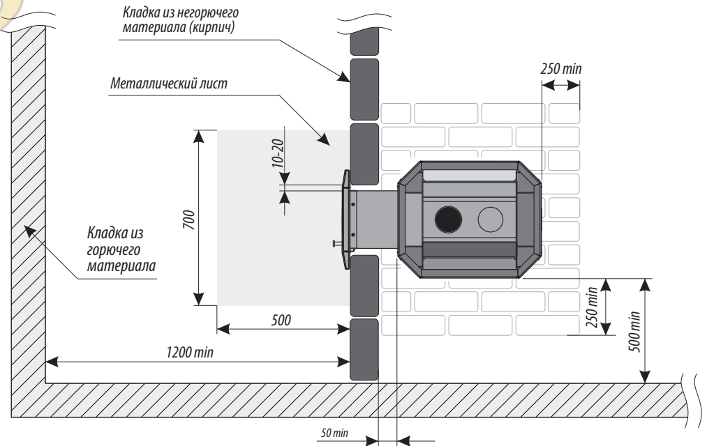
Рисунок 4. Схема установки печи (вид сверху)
