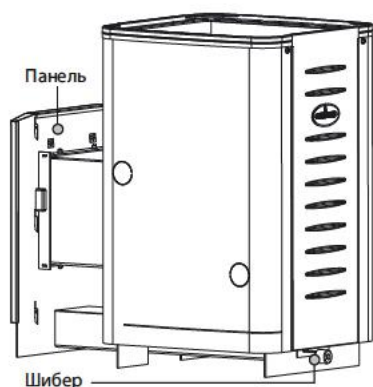
Рисунок 2. Печь Кирасир Стандарт. Вид сзади
