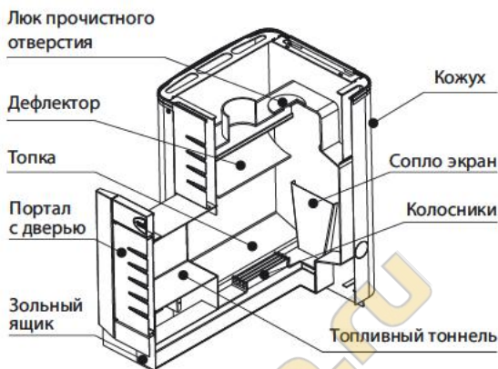
Рисунок 3. Печь Кирасир Стандарт. Вид в разрезе
