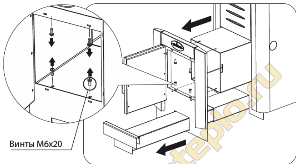
Рисунок 5. Монтаж печи
