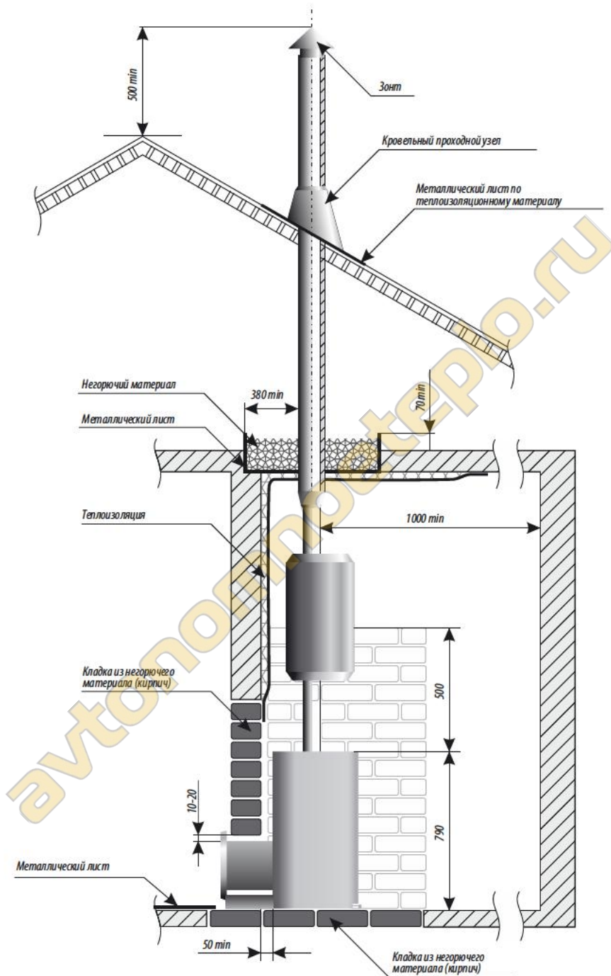
Рисунок 4. Схема установки печи (вид сбоку)
