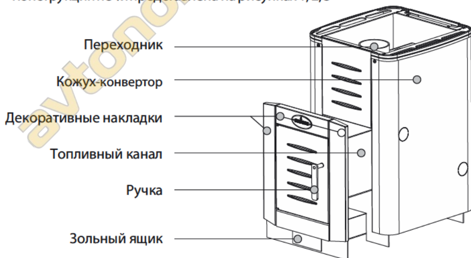
Рисунок 1. Печь Кирасир Стандарт. Вид спереди
