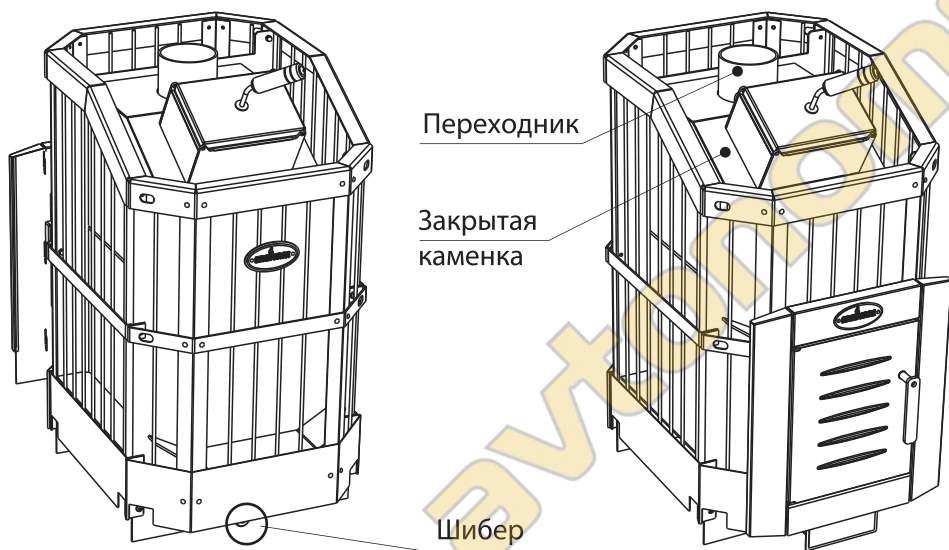
Рисунок 2. Печь Кирасир Атмос Стандарт (вид сзади)
