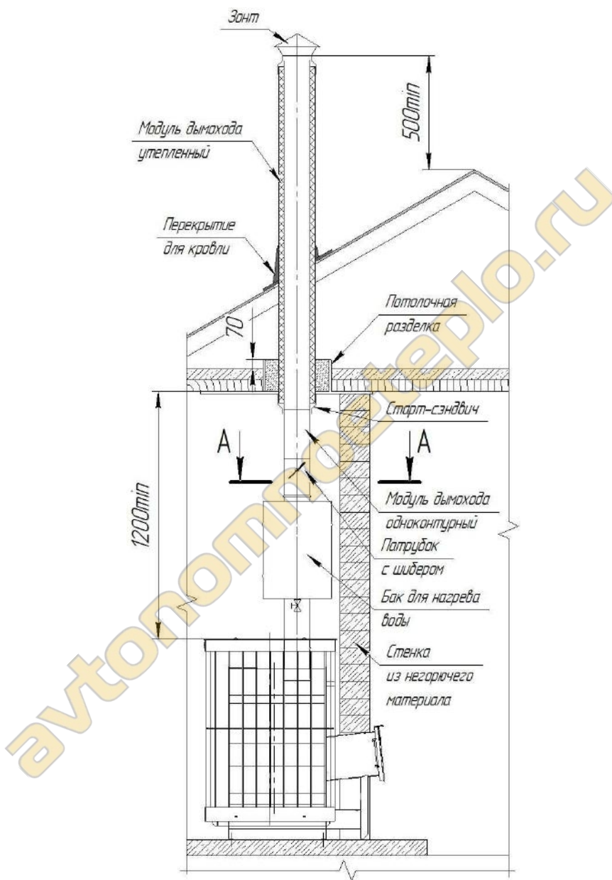
Рисунок 1 – Схема монтажа печи
