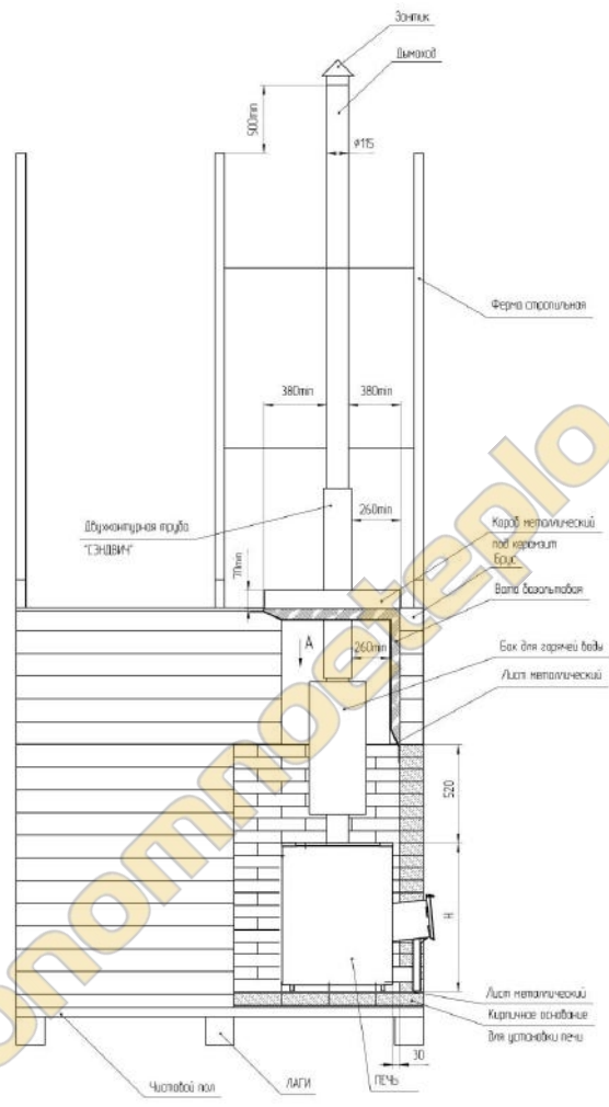
Рисунок 2 – Схема монтажа печи
