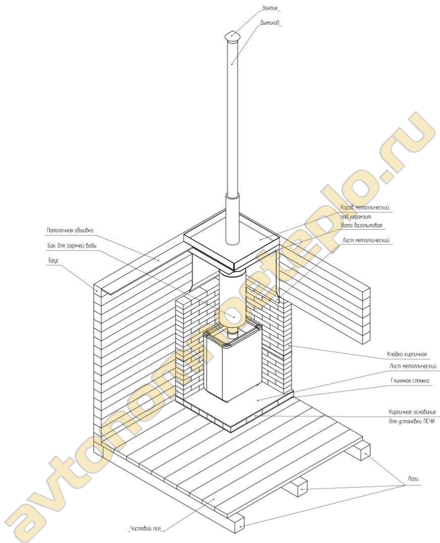
Рисунок 1 – Схема монтажа печи
