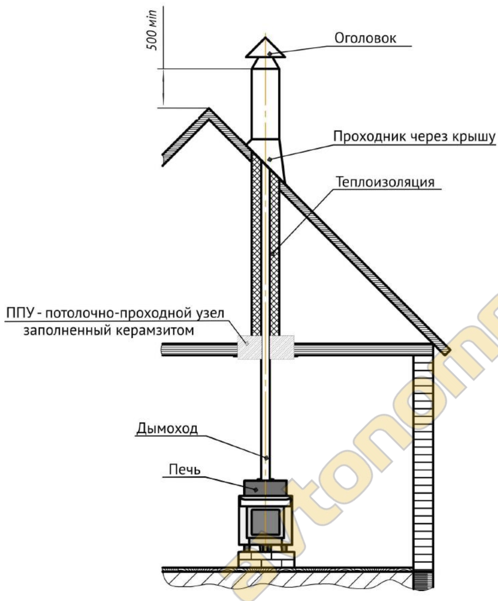
Рисунок 8.6. Монтаж дымового канала.
