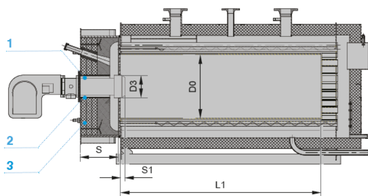
Рис. 5 Установка горелки
