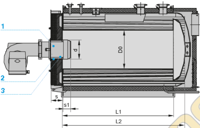
Рис. 5. Установка горелки
