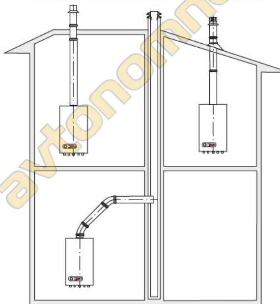
СХЕМА 11 Типы конфигураций монтажа для настенных термических котлов с естественной вытяжкой
