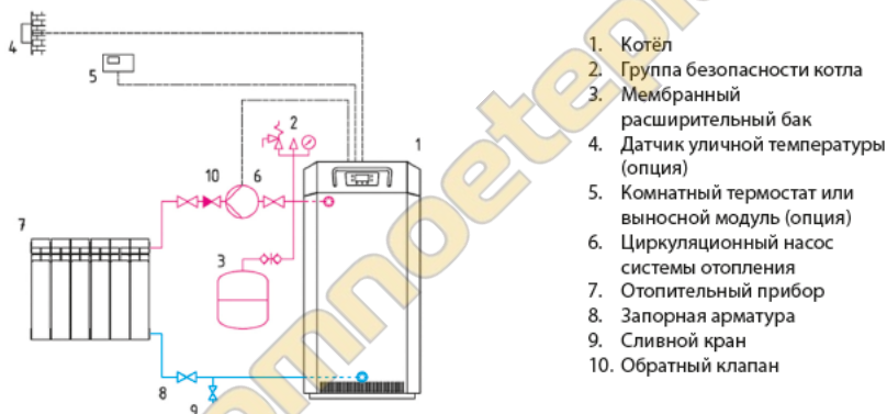
Рис. 6. Гидравлическая схема подключения котла к системе отопления
