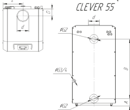
Рис.3. Присоединительные размеры
