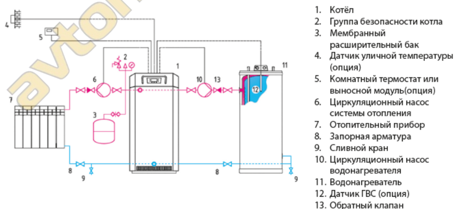
Рис. 7. Гидравлическая схема подключения котла к системе отопления и ёмкостному водонагревателю с двумя насосами
