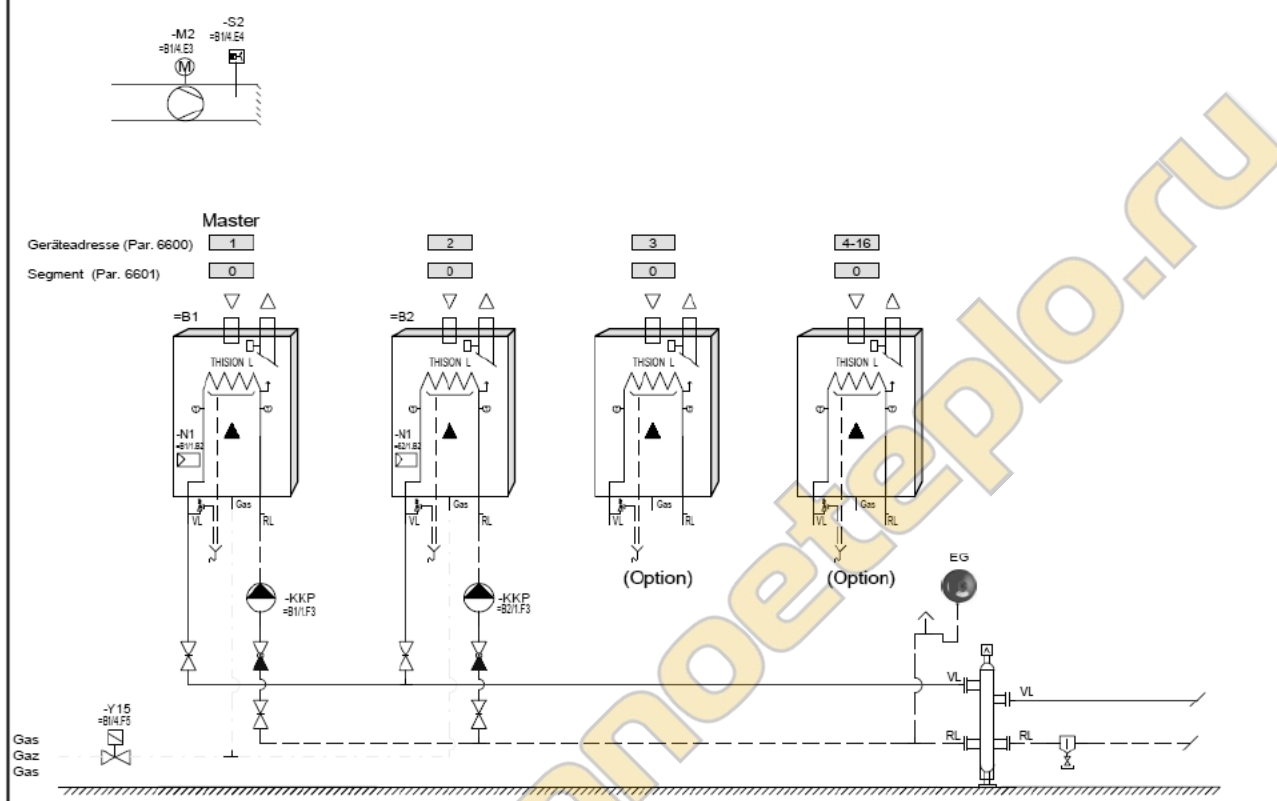
А-С-Е: Система управления через 0-10VDC + каскад через гидравлический разделитель
