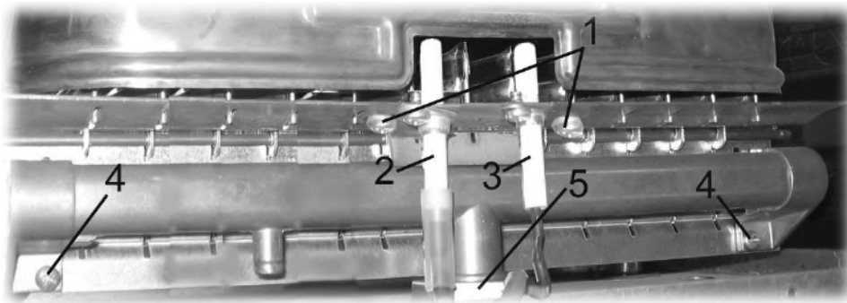
Рис. 17. Демонтаж коллектора
