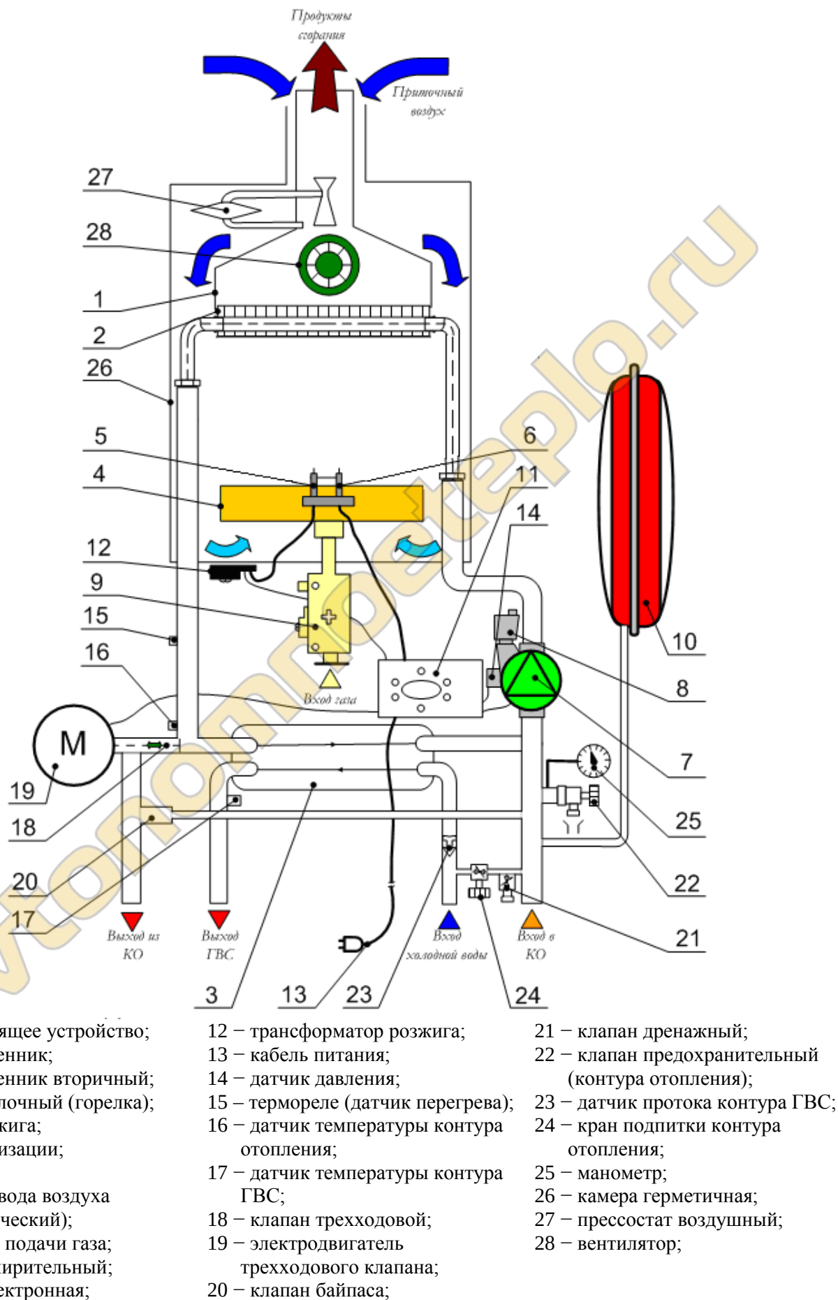
Рис. 14. Функциональная схема котлов «NEVALUX-8224» и «NEVALUX-8230»
