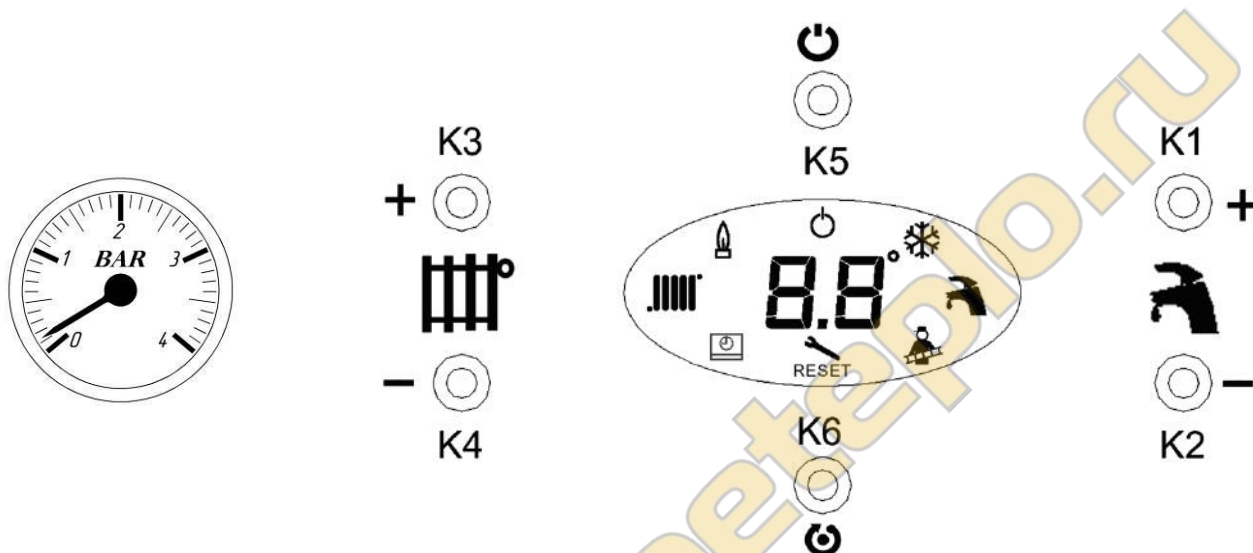
Рис. 3. Панель управления котлом
