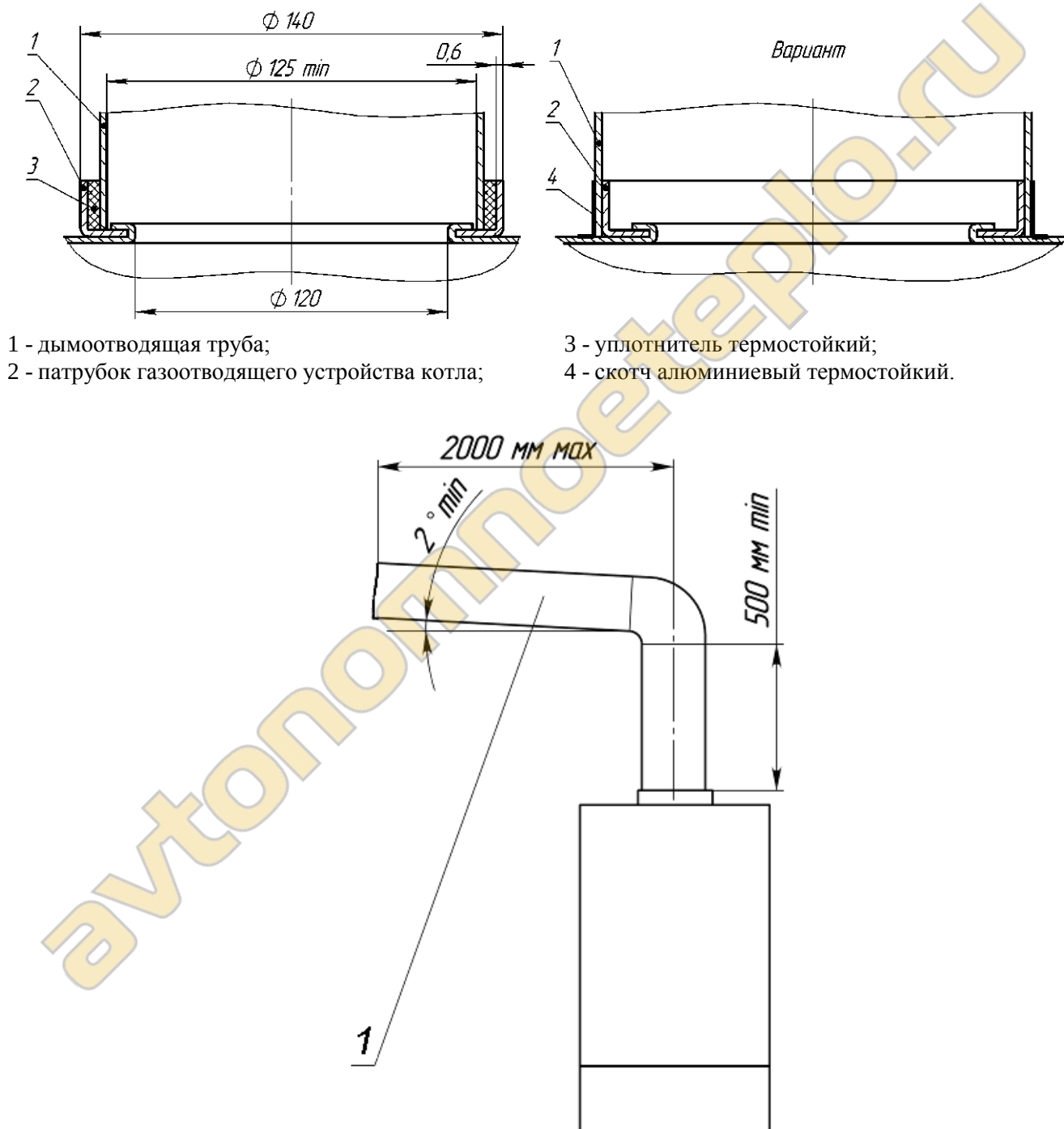
Рис. 11. Схема подсоединения дымоотводящей трубы для котла «NEVALUX-8624»
