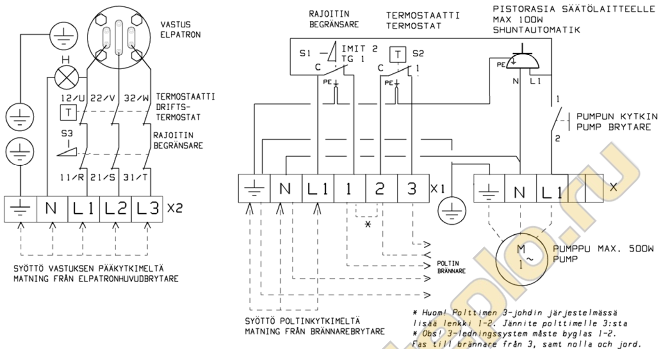
Рис. 2 Схемы электроподключения
