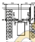
Воздухозабор через стену, дымоотвод в дымоход
