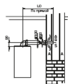
Горизонтальный коаксиальный дымоход
