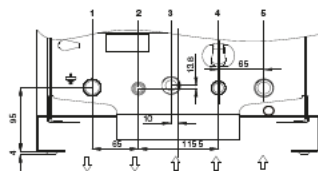
Гидравлические подсоединения
