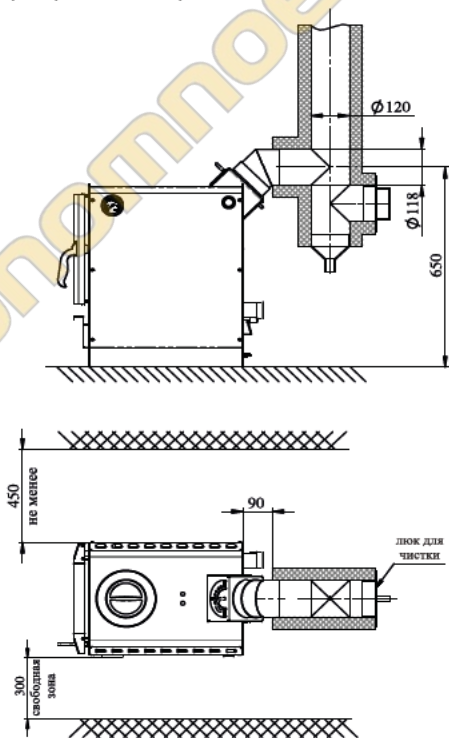
Рис.2 Схема установки аппарата
