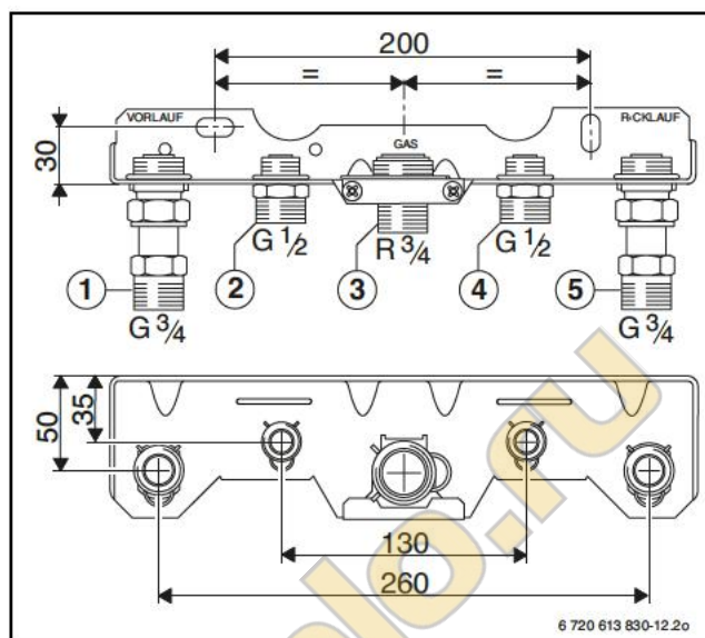
Рис 6 Монтажная панель (дополнительное оснащение)
