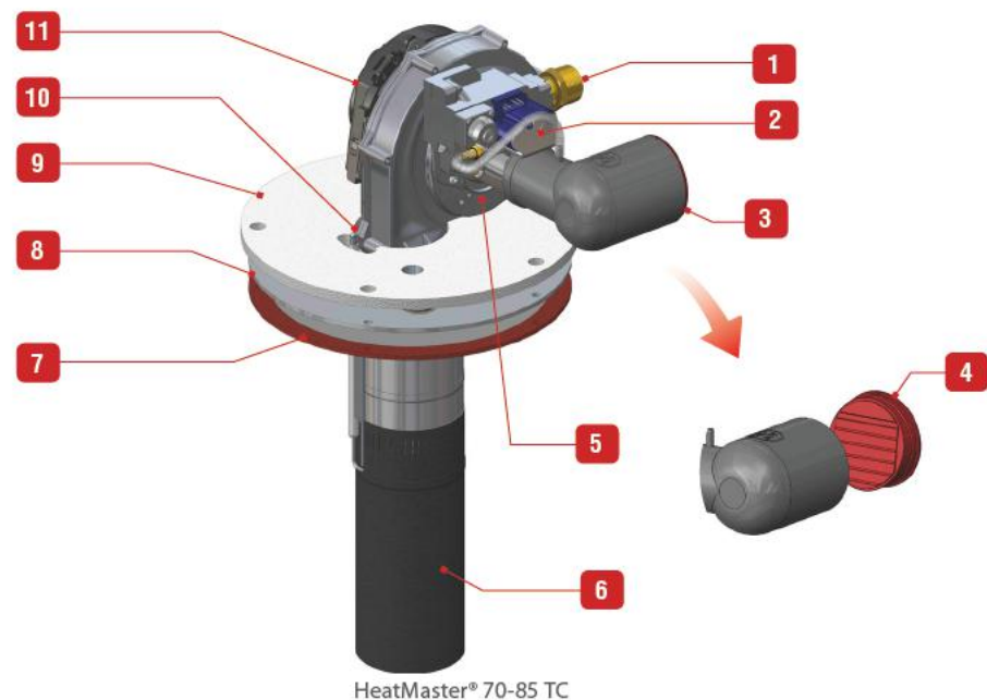
HeatMaster® 70-85 TC
