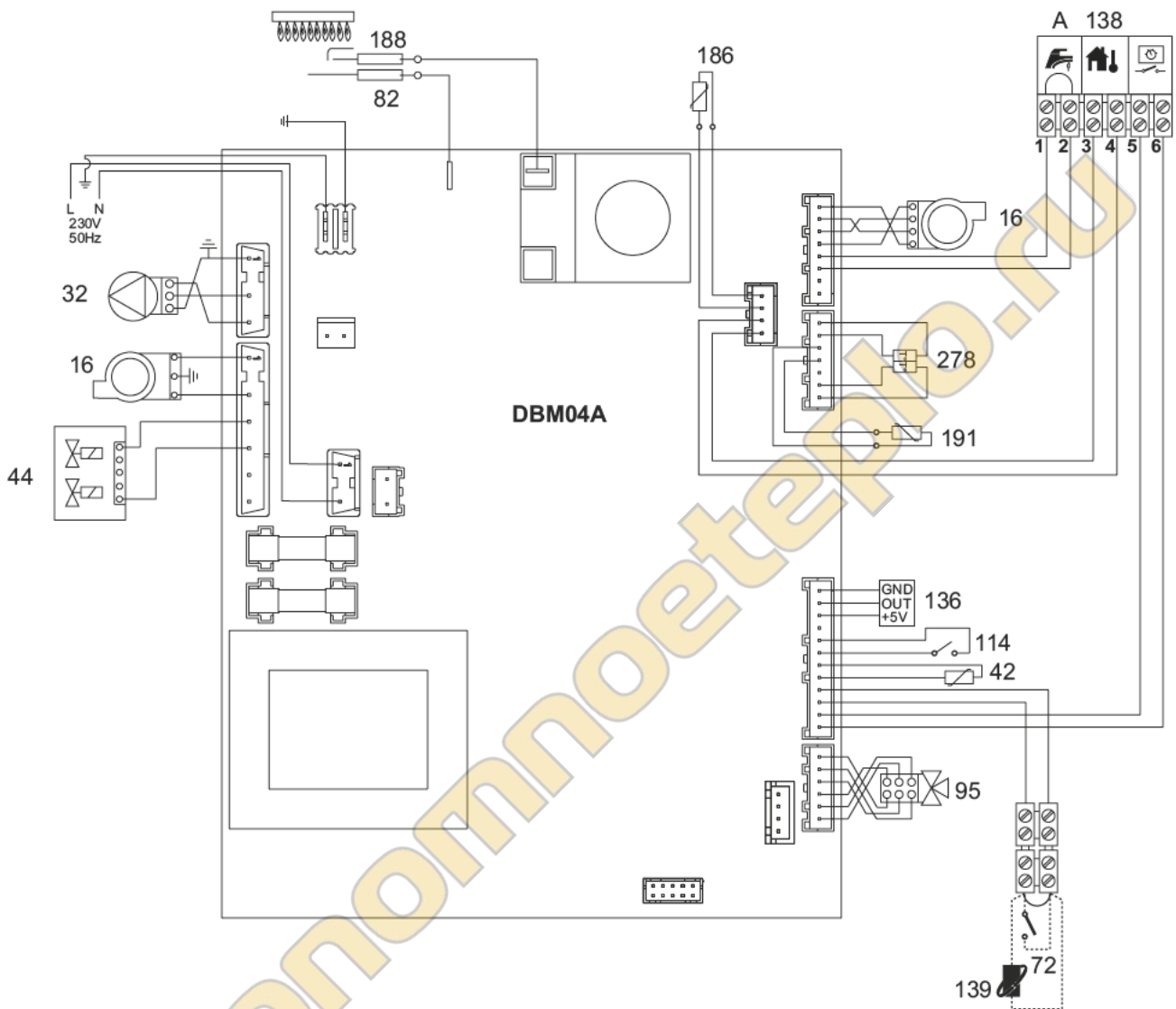
рис. 33 - Электрическая схема
