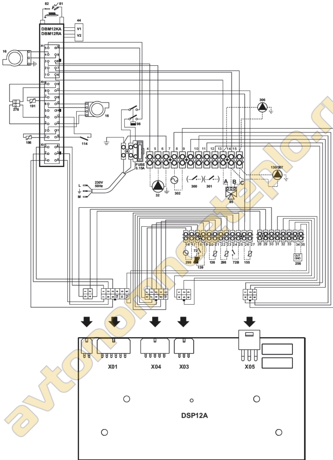
рис. 42 - Электрическая схема
