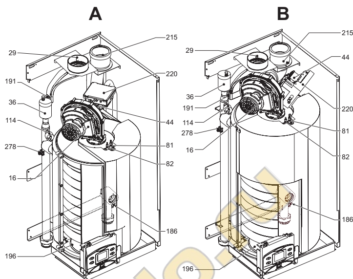
рис. 39 - Общий вид
