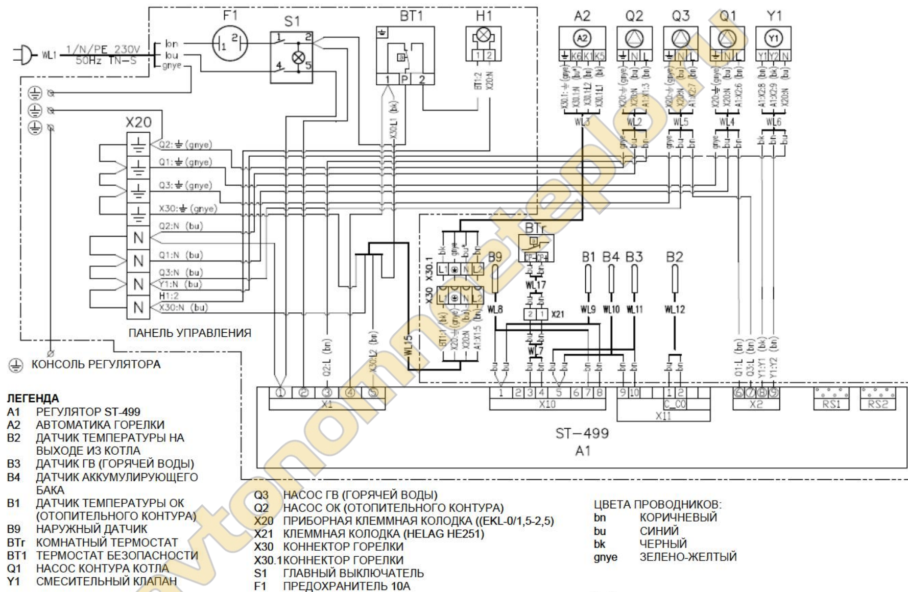
Рис. № 17а) Схема подключения FANDA
