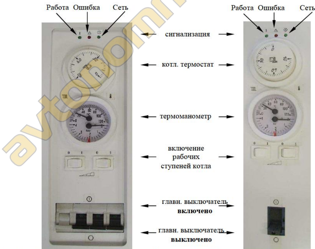
Рис. 30. Панель управления «Daline PTE 4 – 30»
