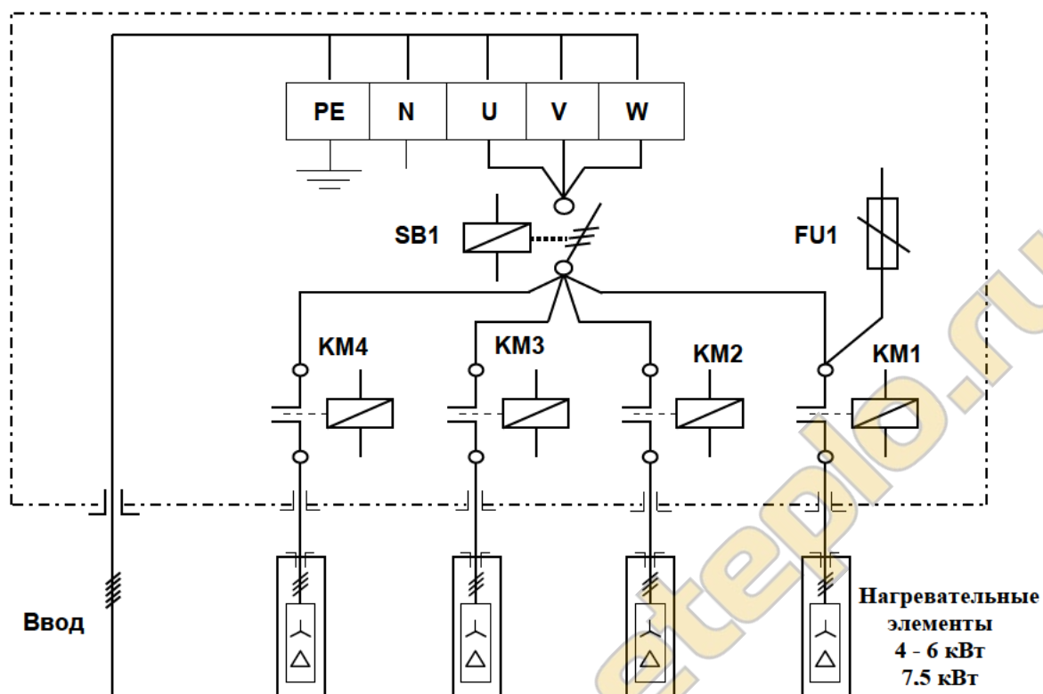
Рис. 9. Силовая схема электрокотла «Daline PTE 22 – 30»
