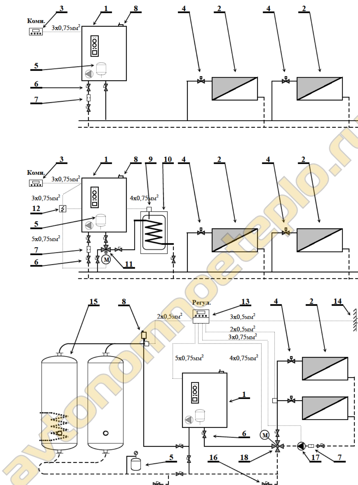
Рис.29. Пример подключения электрокотла к отопительной системе
