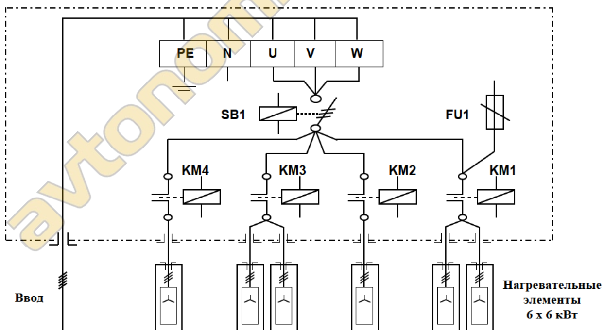
Рис. 10. Силовая схема электродвигателя «Daline PTE 36»
