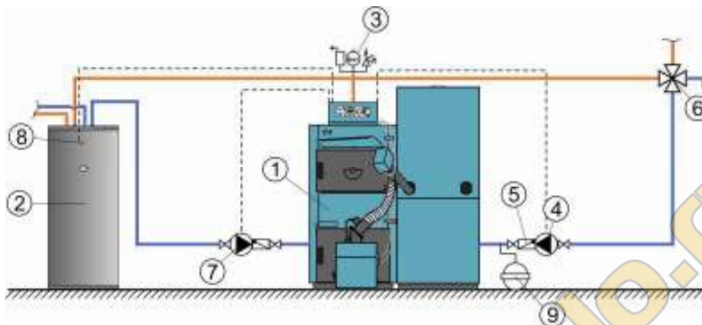
Рисунок 1а. Схема подключения котла ЕКО-СК Р / ЕКО-СКВ Р (ЕКО-СК / ЕКО-СКВ) со встроенным Cm Pelet-набором на установку обогрева со встроенным резервуаром санитарной воды:
