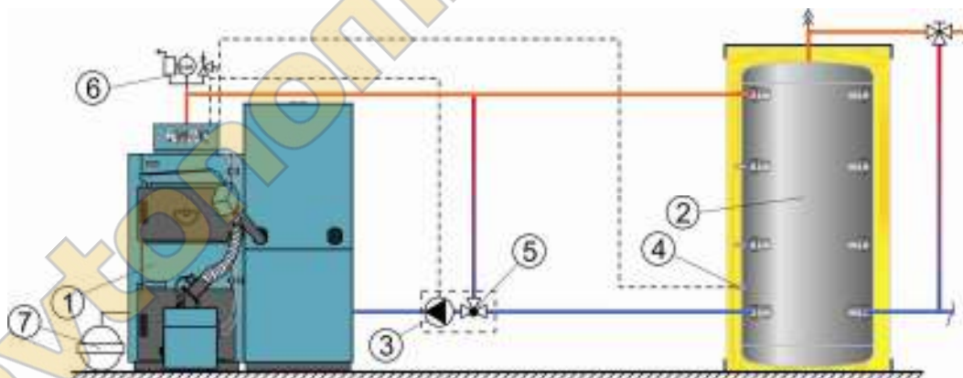
Рисунок 1б. Схема подключения котла ЕКО-СК Р / ЕКО-СКВ Р (ЕКО-СК / ЕКО-СКВ) со встроенным Cm Pelet-набором на установку обогрева со встроенным буферным накопителем (CAS):
