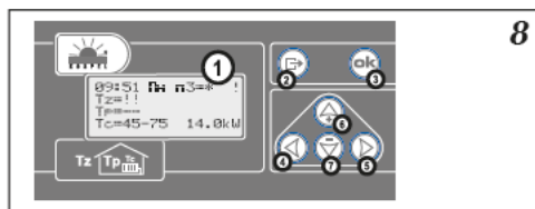
Рис.8 Панель управления ЕКСО.М12/ ЕКСО.ТМ 1 - дисплей, 2-7 - клавиатура
