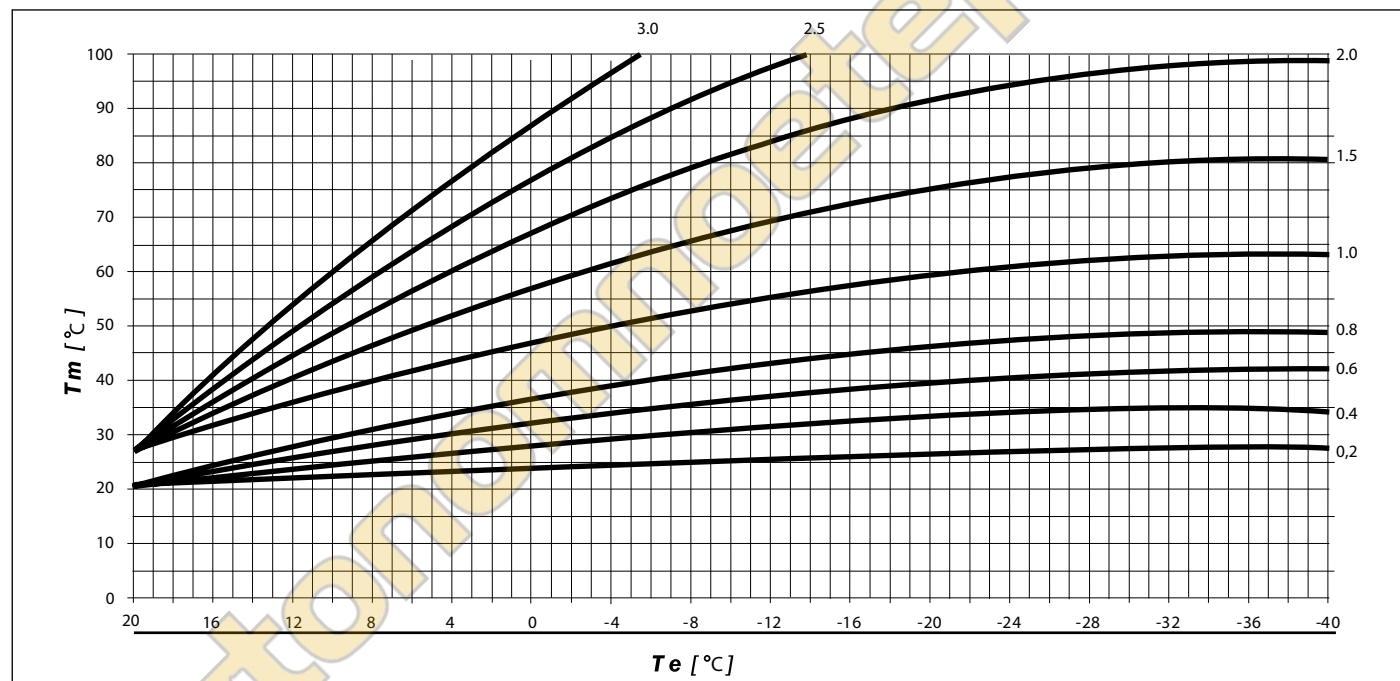
Рис. 14 Температурные кривые
