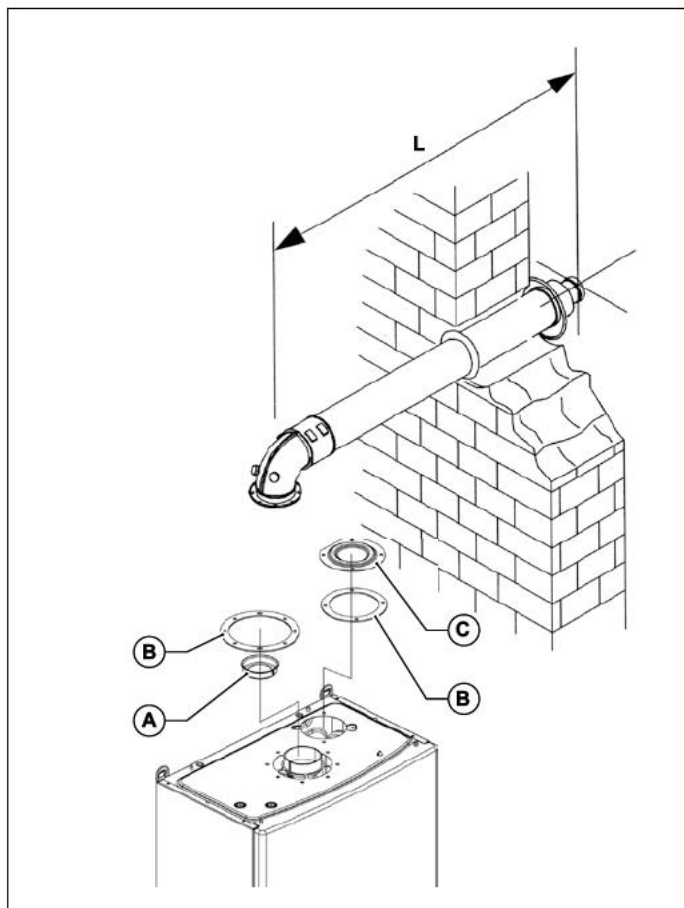
Рис. 6 KITCONC00 (100/60 мм)
