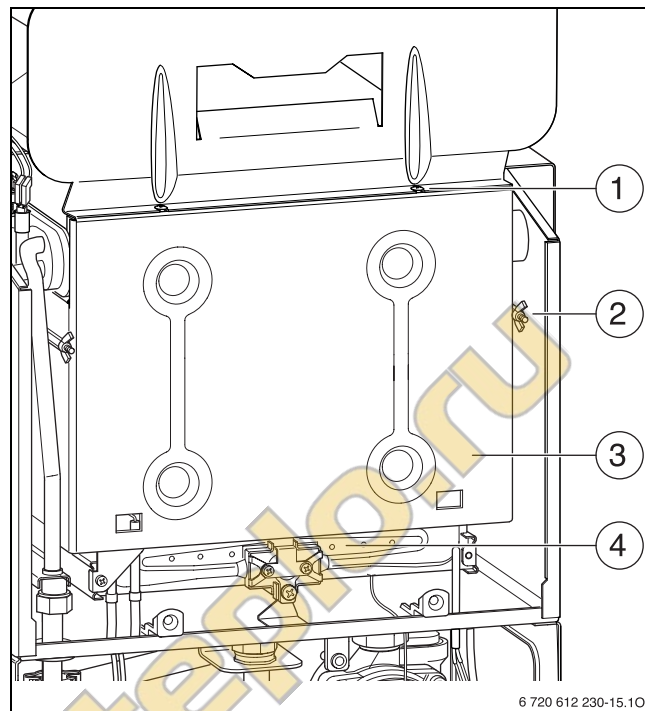
Рис 71 Открывание горелки
