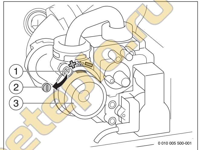
Рис. 47 Регулировка соотношения газ-воздух
