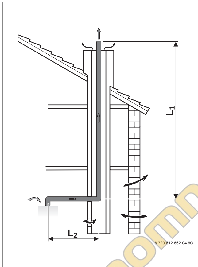
Рис. 8 Дымовая труба в шахте по В 23
