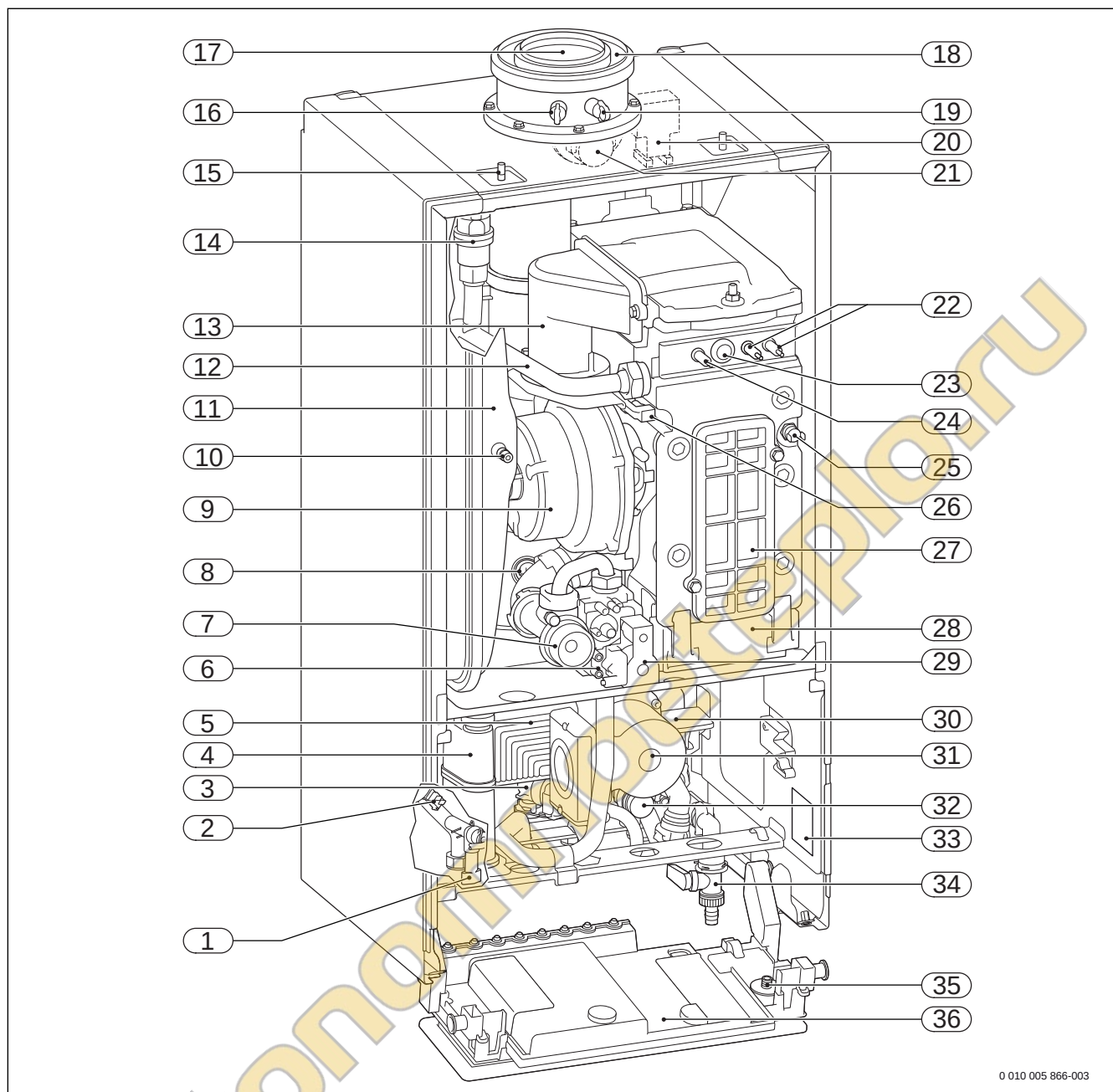
Рис. 3 Обзор GB172i-... K
