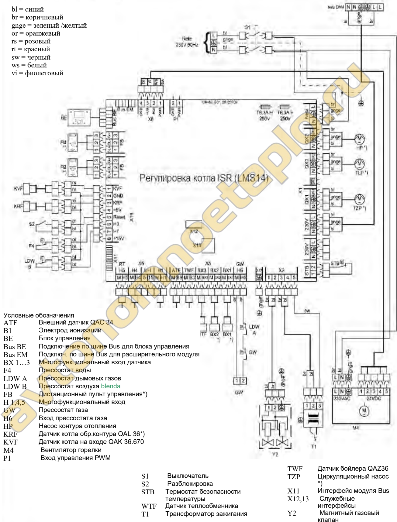
Рис.3. Электрическая схема
