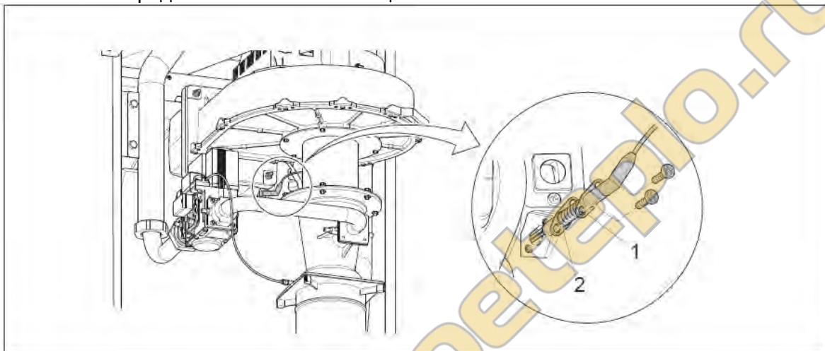
Рис.54. Замена электрода зажигания и ионизации
