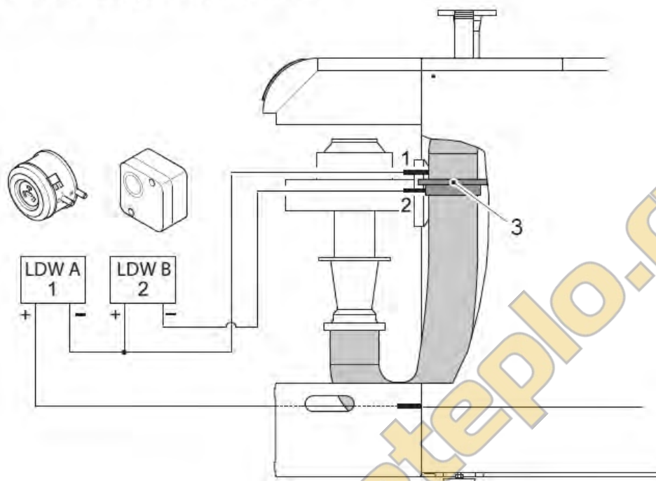
Рис.27. Схема работы воздушного прессостата
