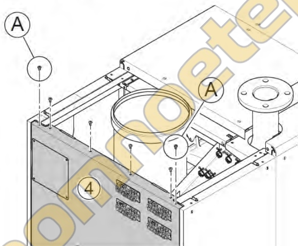
Рис.21. Ослабить верхние крепежные винты
