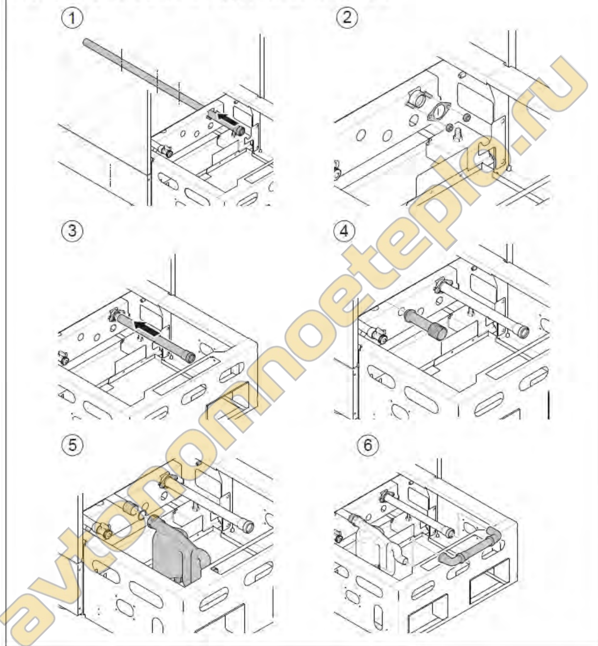
Рис.18. Установка сифона и трубок слива конденсата
