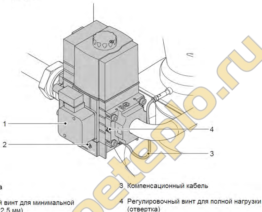
Рис.29. Газовый клапан (Dungs)
