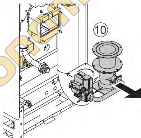
Рис.14. Ослабить трубку Вентури с газовым клапаном
