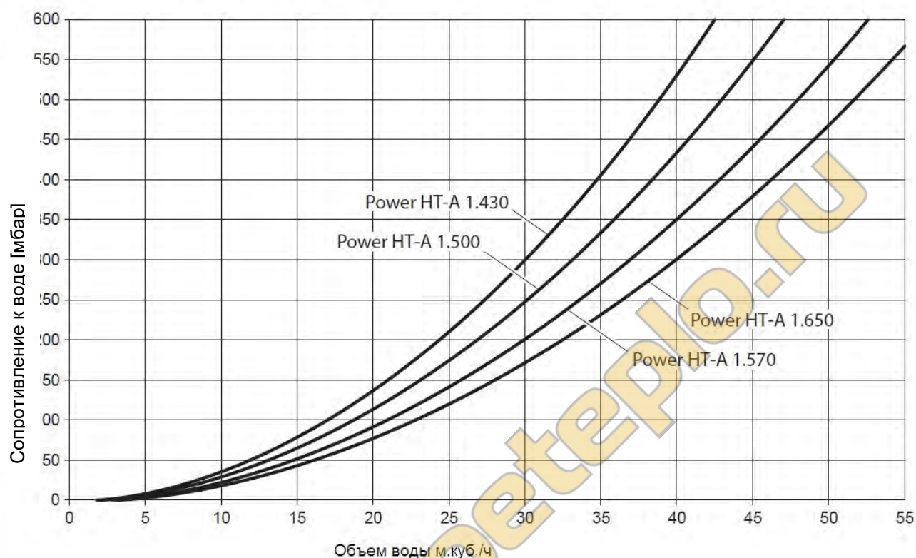
Рис.2. Сопротивление в контуре ГВС Power HT-A 1.430-1.650
