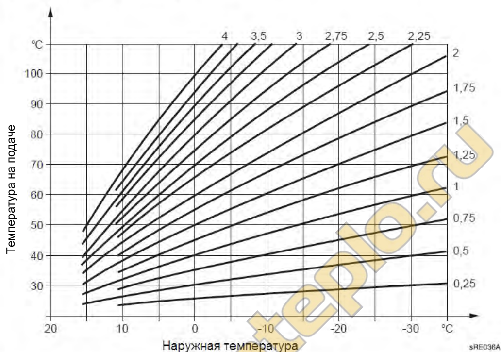
Рис.34. Диаграмма кривых отопления
