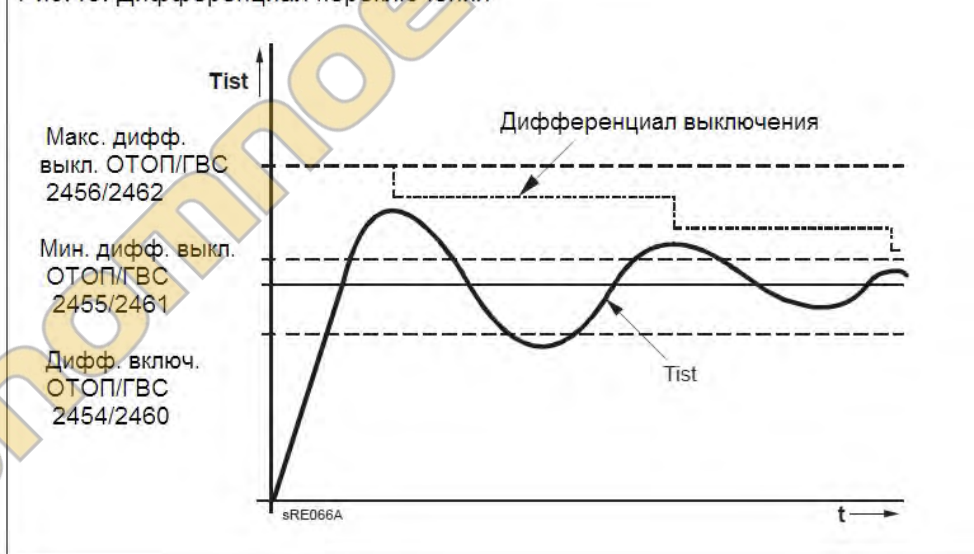
Рис.43. Дифференциал переключения
