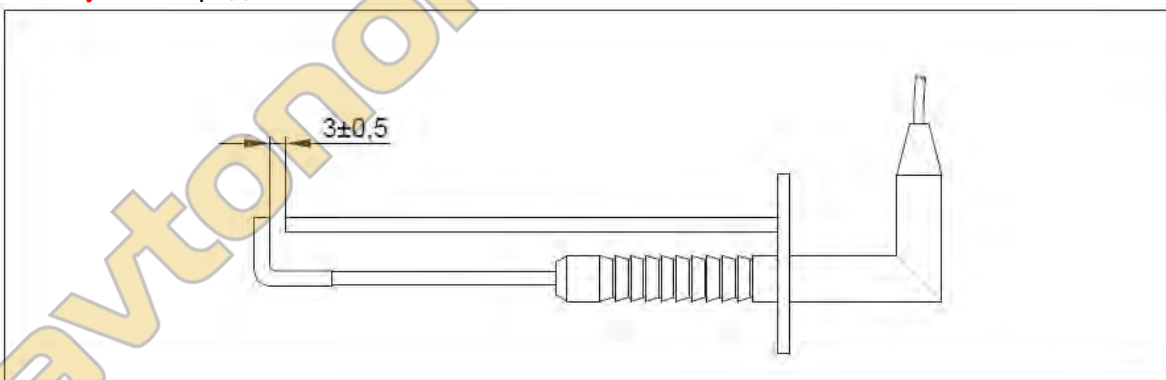
Рис. 55. Выступ электрода
