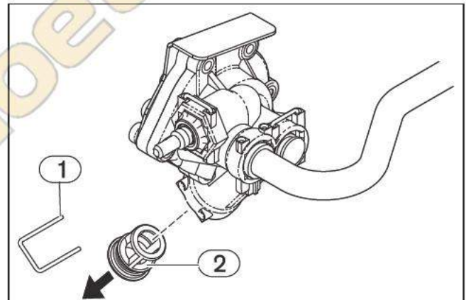
Рис 11 Опорожнение прибора
