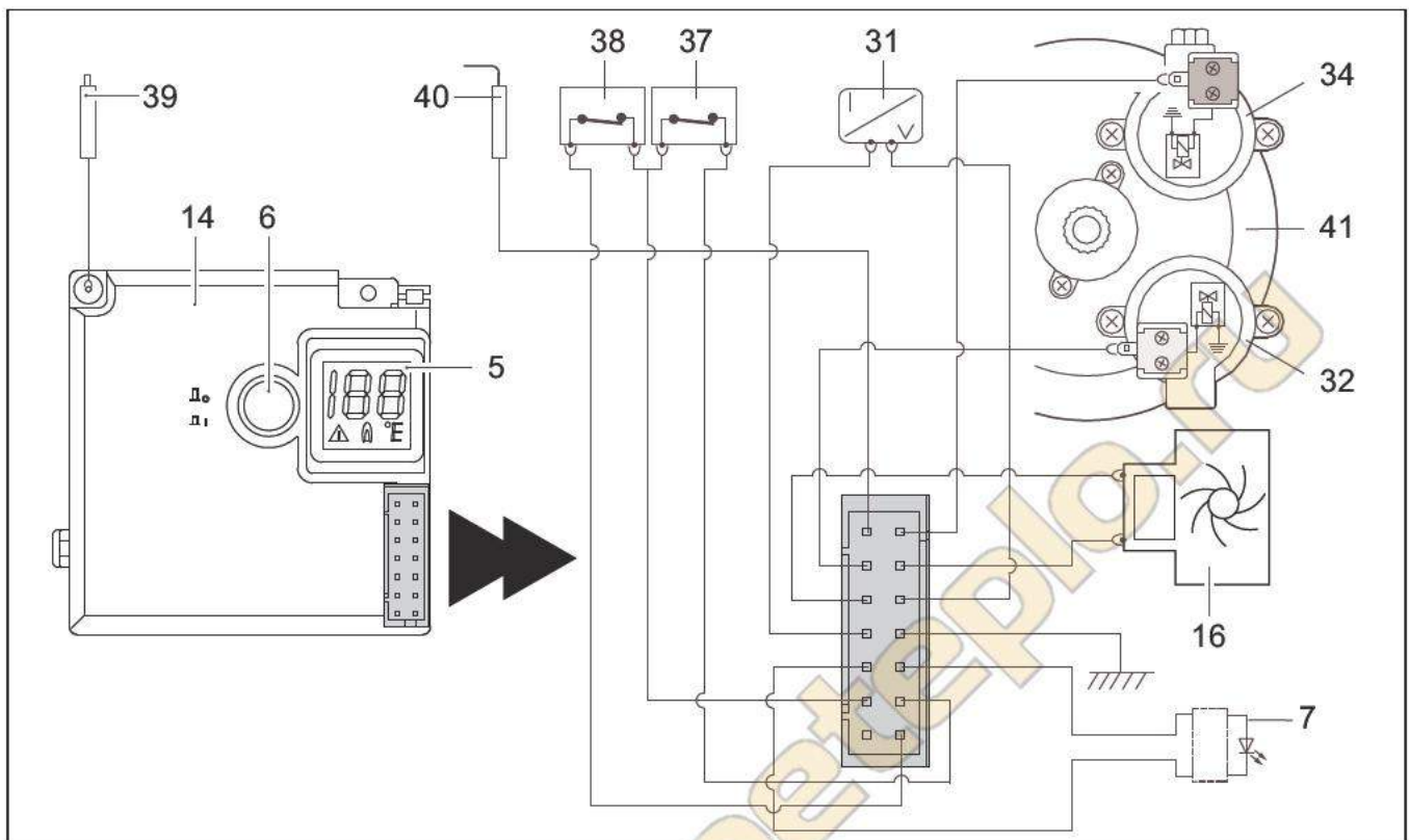
Рис 3 Электросхема
