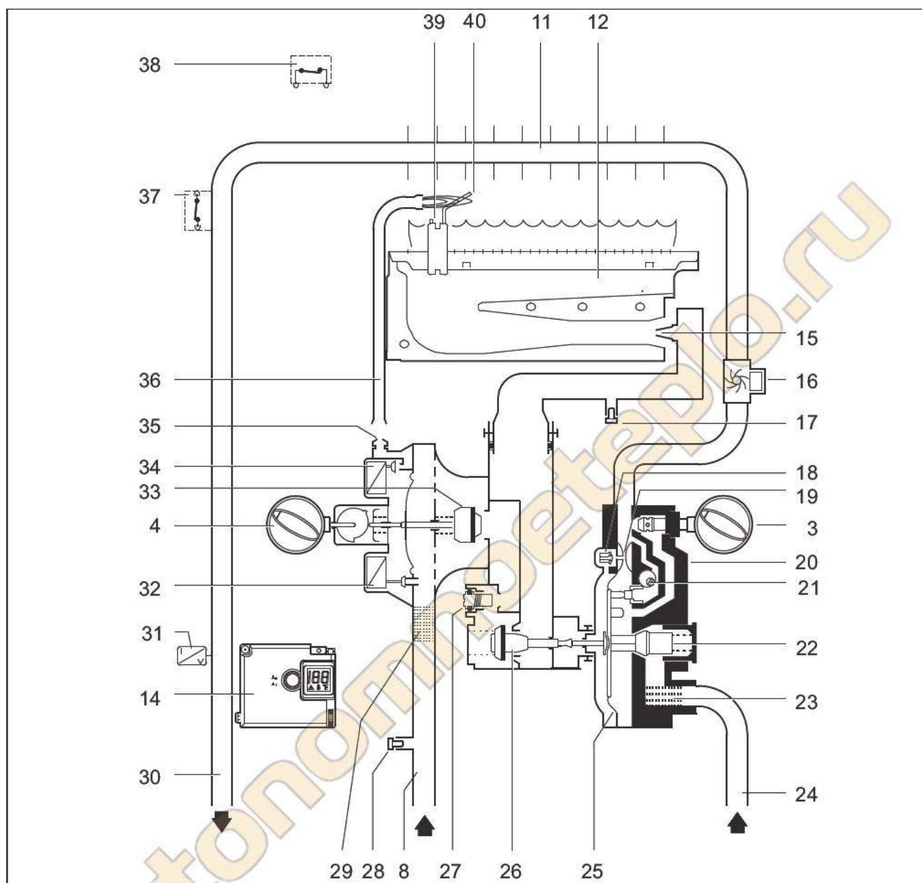
Рис 2 Функциональная схема
