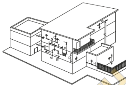
Расположение терминалов для аппаратов с принудительной тягой в зависимости от их теплопроизводительности
