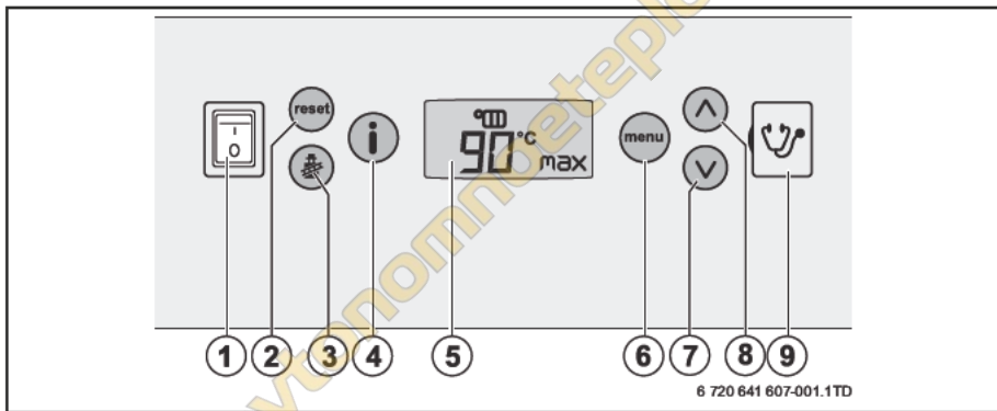
Рис 1 Элементы управления
